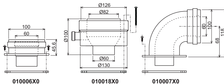
рис. 10 - Элементы для коаксиальных воздухопроводов
