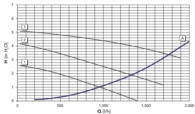
рис. 19 - Потери напора циркуляционных насосов DOMproject F 24 D
