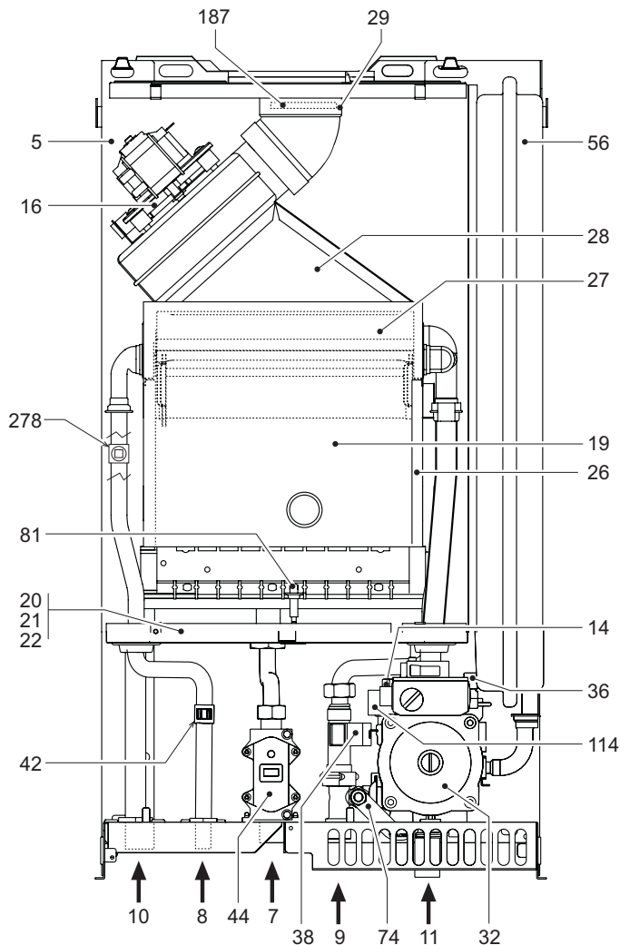
рис. 17 - Общий вид
